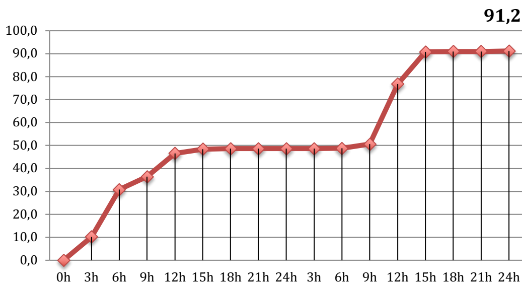
Evolución lluvia acumulada en ALZIRA los días 21 y 22/01/20 en períodos de 3 horas (en l/m 2 )
